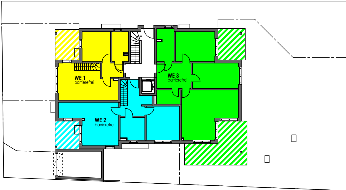
Erdgeschoss
