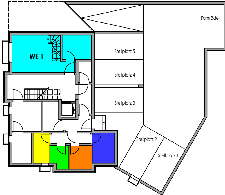
Erdgeschoss
